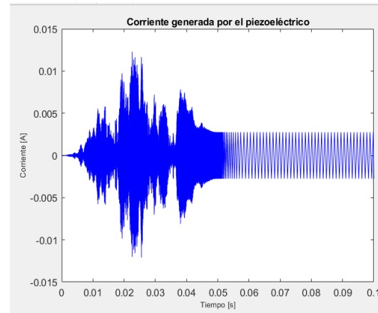
Figura 2: Corriente Generada por un Piezoeléctrico
