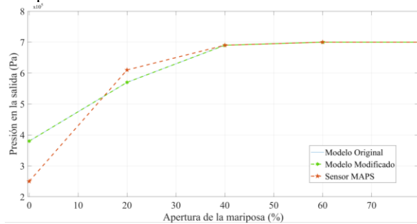
Figura 6: Presiones en la Salida con Diferentes Ángulos de Apertura de Mariposa
