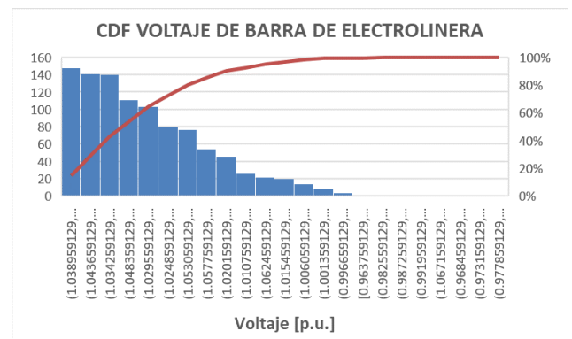
Figura 19: CDF de voltaje de la barra de electrolinera. Caso 2
