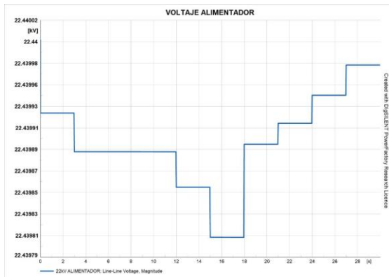
Figura 10: Voltaje del alimentador primario-Condiciónes iniciales
