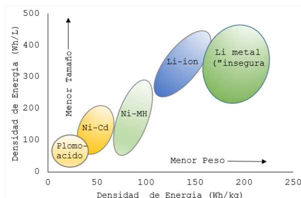
Figura 1: Densidad de energía gravimétrica y volumétrica de diferentes tipos de tecnología de baterías recargables [9]
