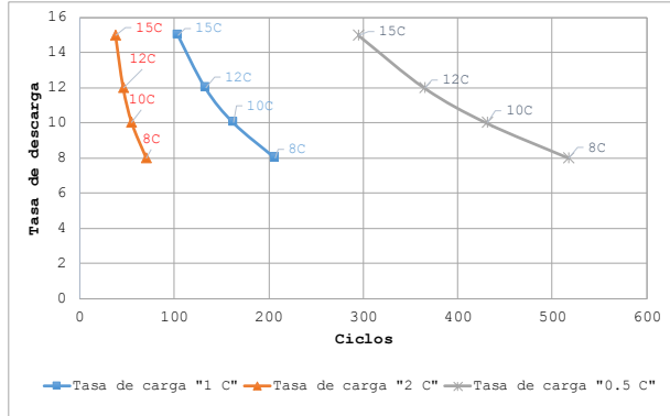
Figura 7: Carga y descargas rápidas de baterías de ion-litio
