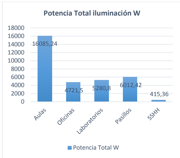
Figura 3: Potencia instalada en iluminación
