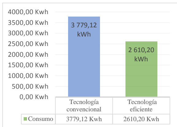
Figura 8. Comparativa de la tecnología convencional con la tecnología eficiente
