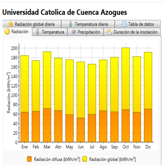
Figura 2: Radiación Global [10]
