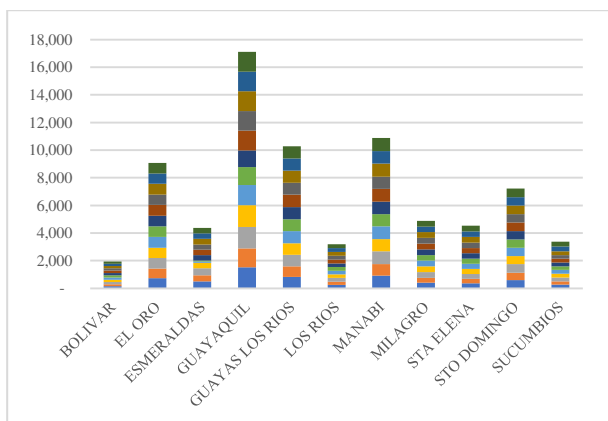
Figura 9. Consumo de auxiliares de CNEL del año 2019 según la propuesta en MWh
