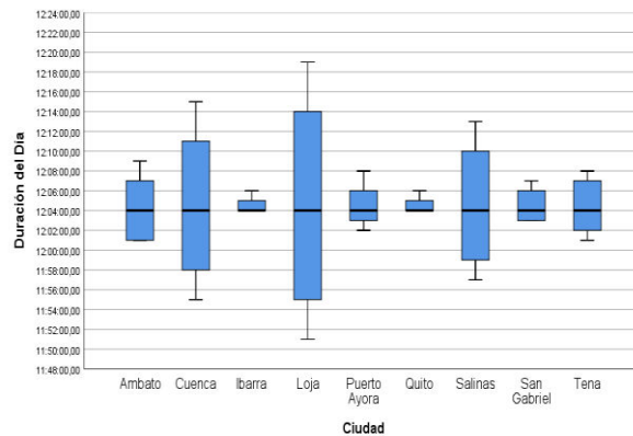
Figura 5: Duración del día por ciudad
