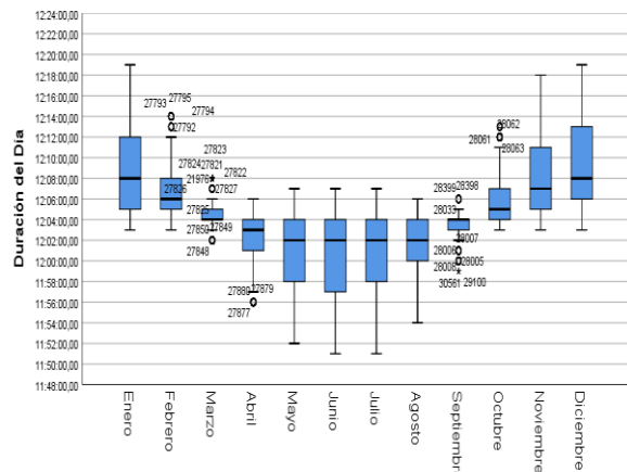
Figura 4: Duración del día por mes
