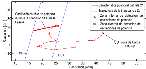
Figura 29: Primera oscilación estable de potencia presente en la fase-B durante la condición SPO de la fase-A
