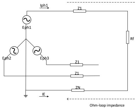
Figura 5: Lazo de medición en fallas monofásicas [2]
