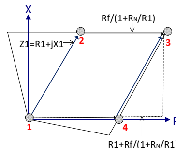
Figura 7: Característica de diseño en ohm-phase del elemento fase-tierra
