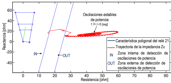
Figura 31: Trayectoria de Zb ante oscilaciones de potencia
