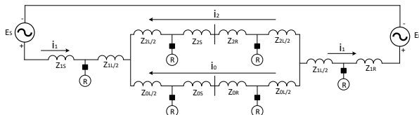
Figura 9: Circuito de redes de secuencia negativa y cero
