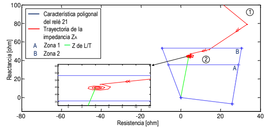
Figura 23: Efecto de sub-alcance en la trayectoria de la impedancia Z_a
