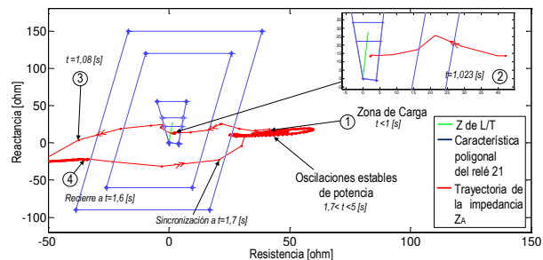
Figura 26: Trayectoria de Z_a vista por R-21S en presencia del esquema SPS
