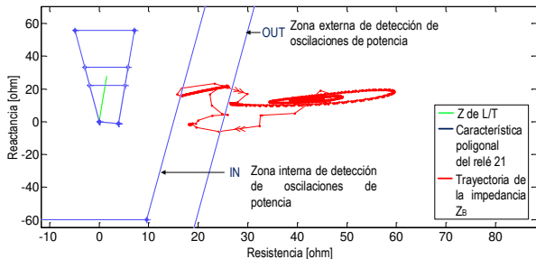
Figura 28: Trayectoria de Z_b en presencia del esquema SPS para la fase-A
