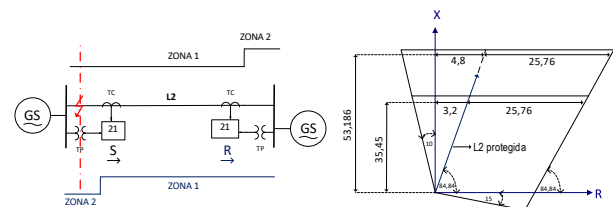
Figura 15: Configuración de los R-21 ubicados en S y R
