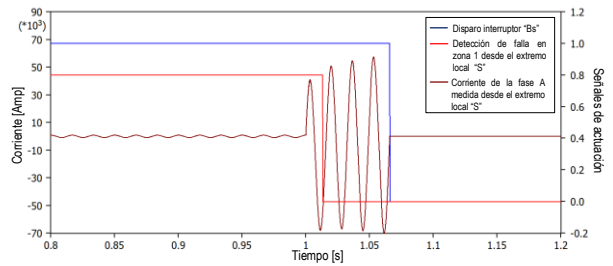
Figura 16: Detección de falla y disparo desde el extremo S
