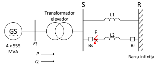
Figura 13: Modelo de simulación del SEP de prueba [3]
