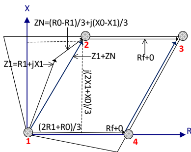
Figura 6: Característica de diseño en ohm-loop del elemento fase-tierra
