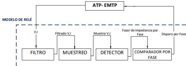
Figura 11: Estructura de modelamiento del relé de distancia en ATP
