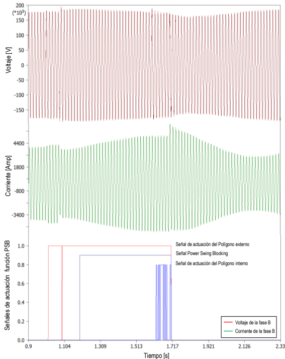
Figura 32: Detección de oscilaciones estables de potencia mediante el método convencional de tasa de cambio de la impedancia
