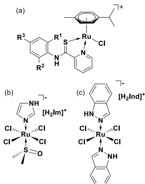
Figura 4: (a) Areno(piridino-carbotioamida)rutenio(II). (b) NAMI-A: (H 2 im)( trans -RuCl 4 (Him)(dms)) (Him=imidazol, dms=dimetil sulfóxido). (c) KP1019: (H 2 Ind)( trans -(tetraclorobis(HInd)rutenato(III)) (HInd=1H-indazol).
