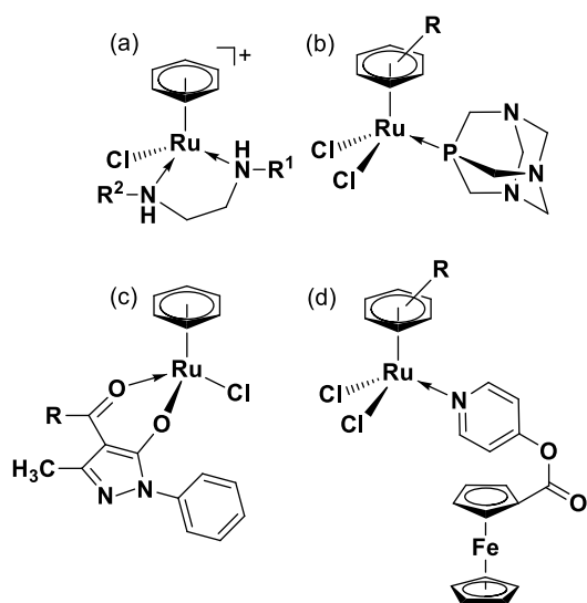
Figura 3: (a) Areno(etilendiamino)rutenio(II). (b) Areno(PTA)rutenio(II) (denominado RAPTA) con PTA = 1,3,4-triaza-7-fosfatriciclo-(3.3.1.1) decano. (c) Areno (acil-pirazolona) rutenio(II). (d) Areno (piridin-monoacetylferroceno) rutenio(II).
