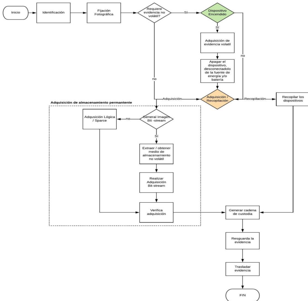
Gráfico 1. Modelo propuesto
