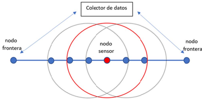
Fig. 1. Red inalámbrica de sensores con topología lineal.
