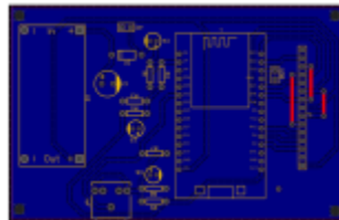
Figura 5. Diseño PCB
