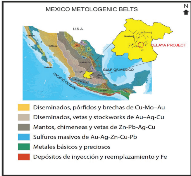
Figura 1. Cinturón de Metalogenia México Fuente: Servicio Geológico Mexicano, 2014
