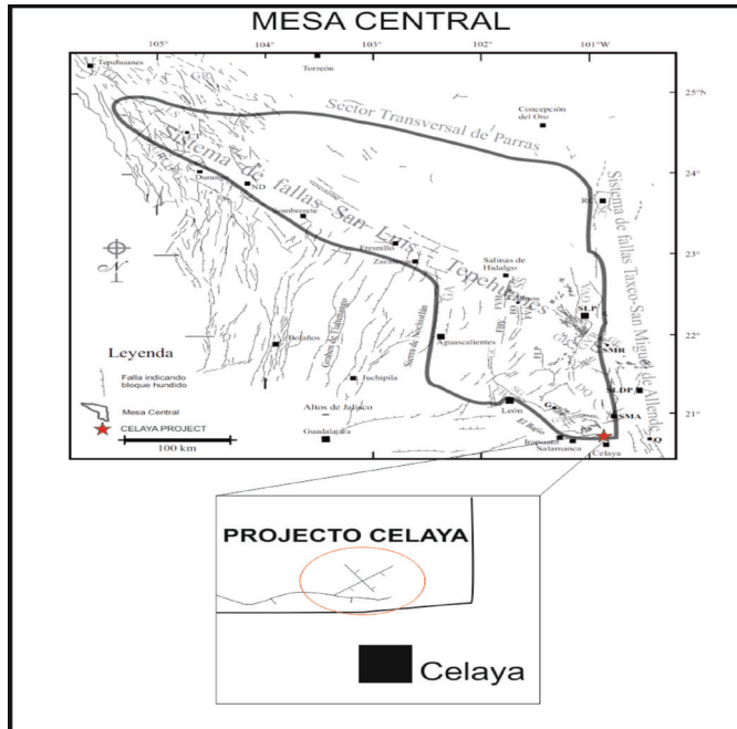
Figura 3. Mapa que muestra la localización de las estructuras de la mesa central.
