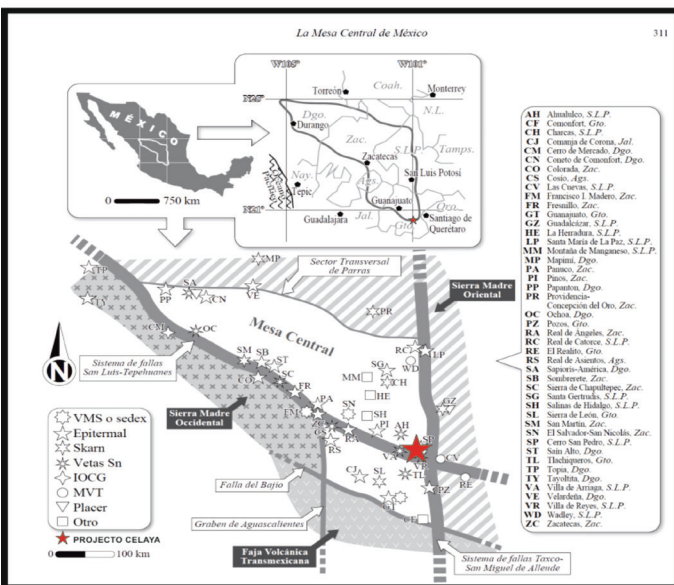
Figura 4. Mapa de la localización de los principales depósitos minerales de la mesa central.
