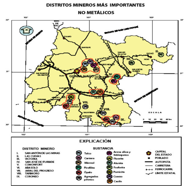
Figura 5. Mapa de minas para no metálicas Guanajuato
