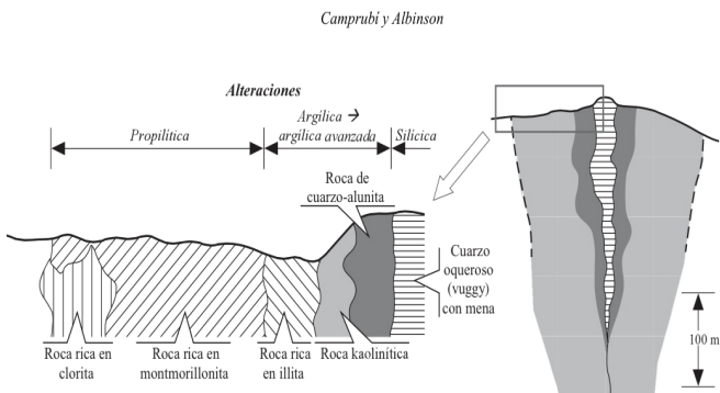
Figura 7. Esquema de Zonamiento-Vectorización de arcilla
