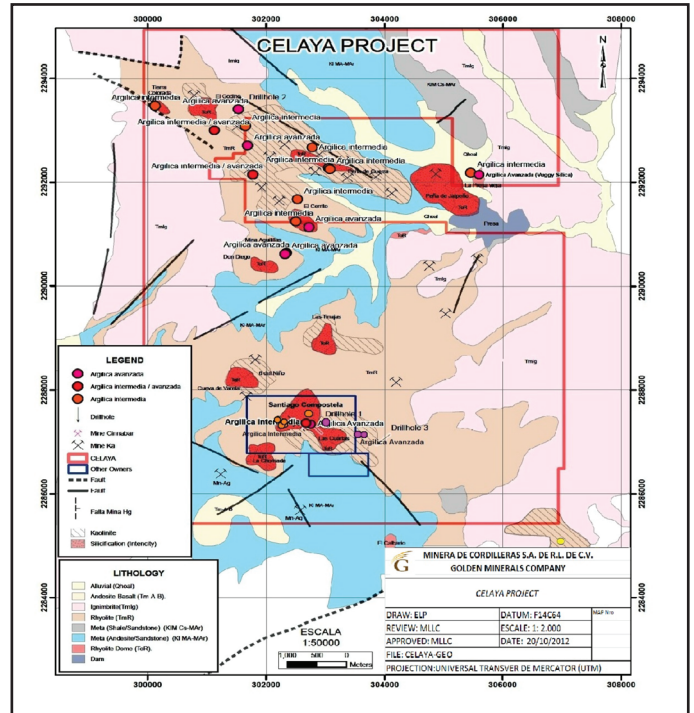
Figura 8. Mapa de Muestreo de Arcillas Vectorización y Zonamiento
