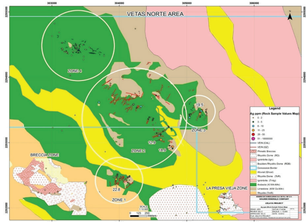
Figura 10. Resultados para Ag vetas norte sector 1
