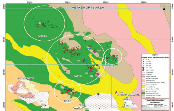
Figura 9. Resultados para Au vetas norte sector 1
