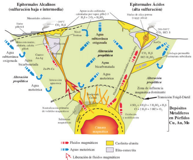
Figura 2. Modelo geológico de sistemas epitermales de alta y baja sulfuración
