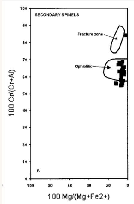
Figura 1. Diagrama Cr-Al/Mg-Fe 2+ , los cristales de espínelas cromíferas parte de las rocas de la zona de cizallamiento Naranjal plotean dentro del campo ofiolítico propuesto por Haggerty (1991) para espínelas secundarias (adaptado de Pilatasig, 2001).
