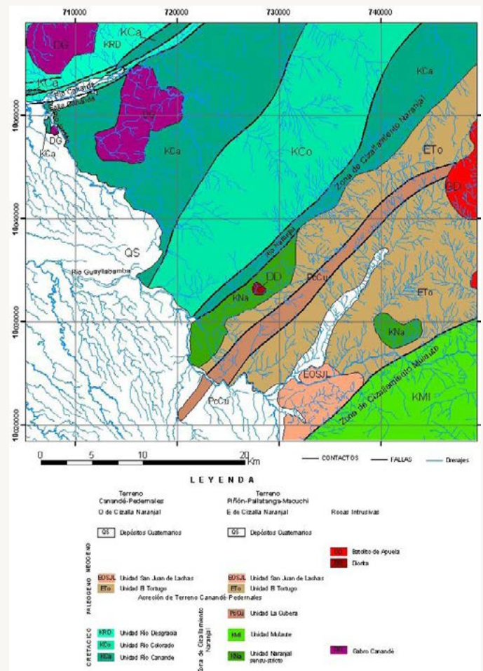
Figura 2.- Mapa geológico de la zona de interés, incluyendo la hipótesis propuesta (Modificado de Boland et al., 2000; y Pilatasig et al., 2004)..
