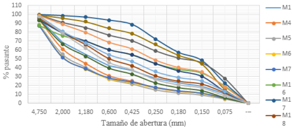
FIGURA 8 Curvas granulométricas de la zona sin intervención
